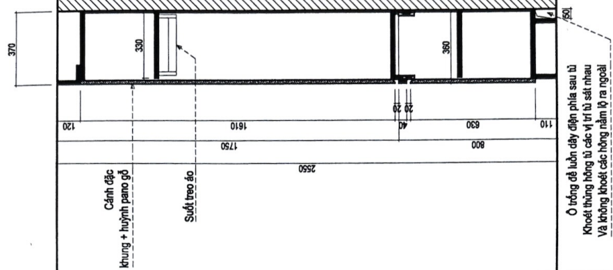
MẶT CẮT 4-4 (TỪ TÀI LIỆU CẢNH ĐẠC 4)
