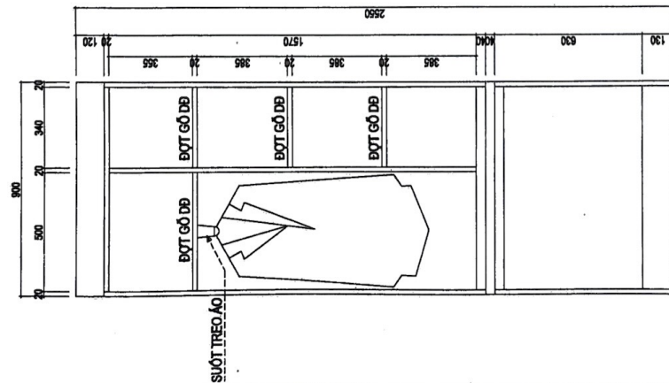
MẶT ĐỨNG BỜ CÁCH (TỦ TÀI LIỆU 4) SL: 01 bộ
