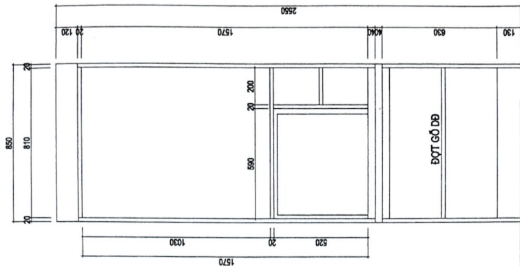
MẶT ĐỪNG BỎ CẢNH ( TỪ TÀI LIỆU 2 - CẢNH GỖ ĐẶC) SL : 01 bộ
