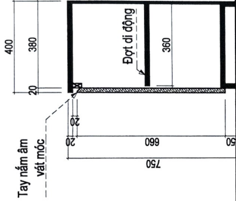
MẶT CẮT
