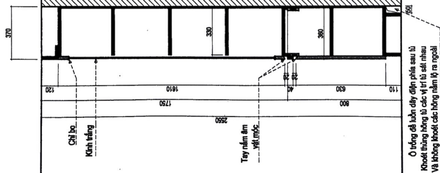
MẶT CÁT 1-1 ( TỪ TÀI LIỆU CẢNH KINH + CẢNH ĐẶC 1 )
