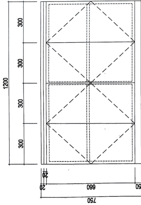
MẶT ĐỨNG
