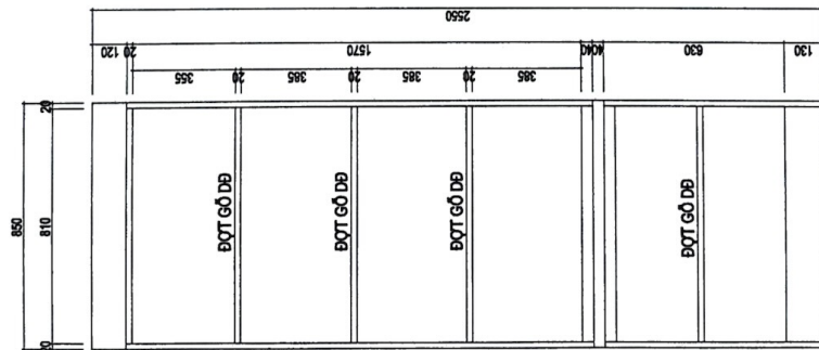
MẶT ĐỨNG BỜ CÁN ĐIỂN HÌNH (TỦ TÀI LIỆU 1 - CÁN KÍNH & GỖ ĐẶC) SL : 10 bộ
