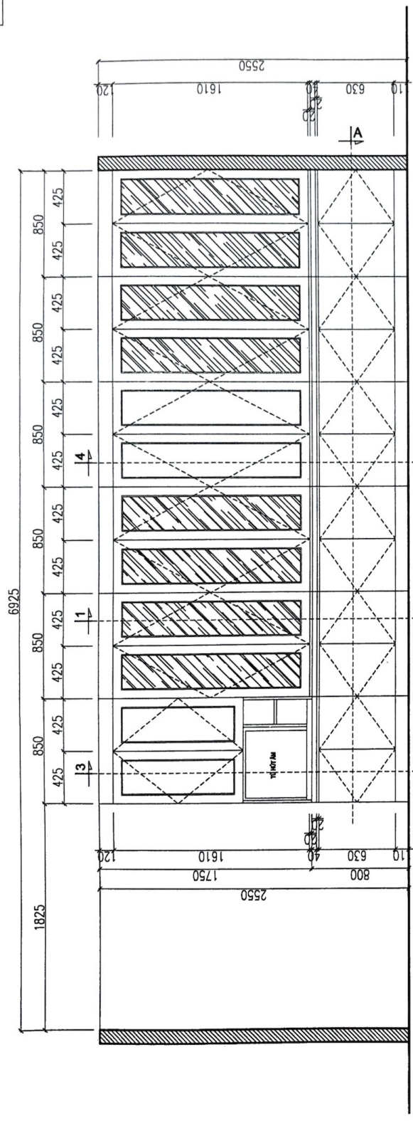
MẶT ĐƯƠNG - HỆ TỦ B
